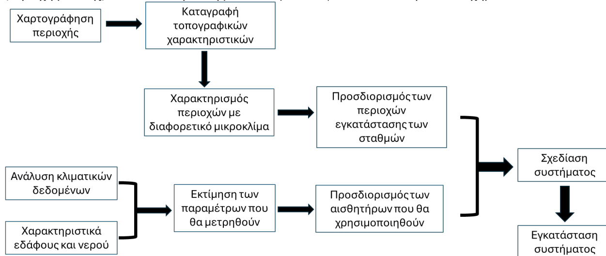
Εικόνα 1. Διάγραμμα της διαδικασίας σχεδιασμού και εγκατάστασης ενός καταναμημένου ασύρματου δικτύου σταθμών
