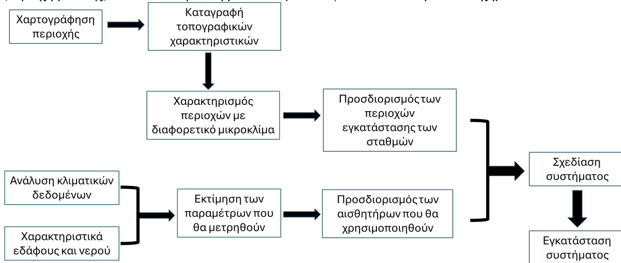
Εικόνα 1. Διάγραμμα της διαδικασίας σχεδιασμού και εγκατάστασης ενός κατανεμημένου ασύρματου δικτύου σταθμών
